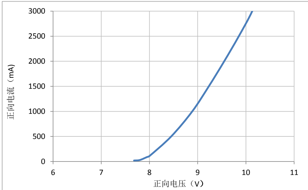
正向电压 vs 正向电流 (环境温度25°C)
