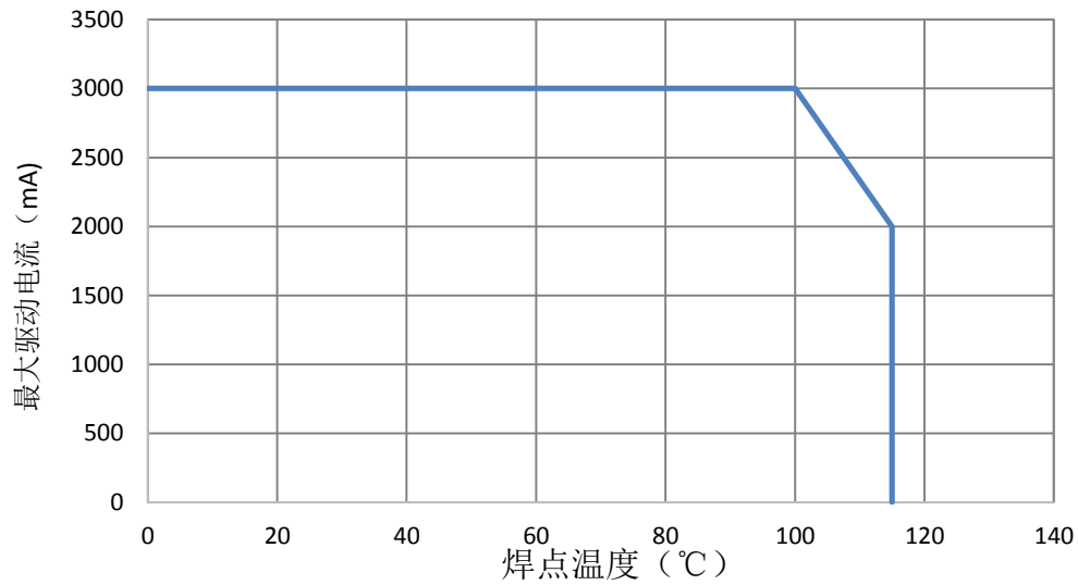
驱动电流 vs 焊脚温度
