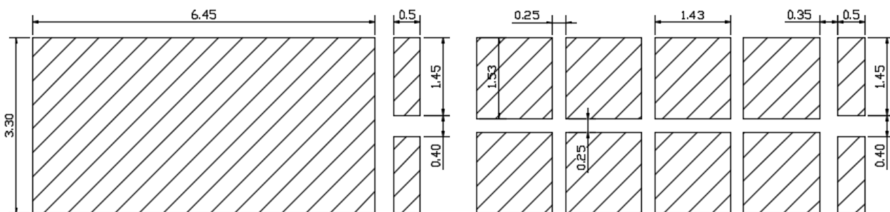
推荐 PCB 焊盘尺寸
