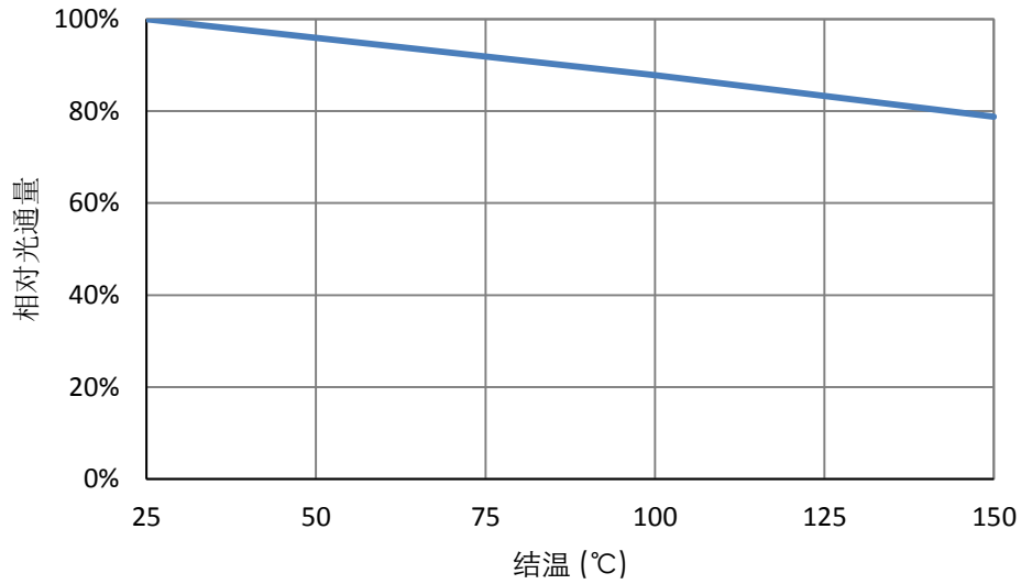
相对光通量 vs 结温
