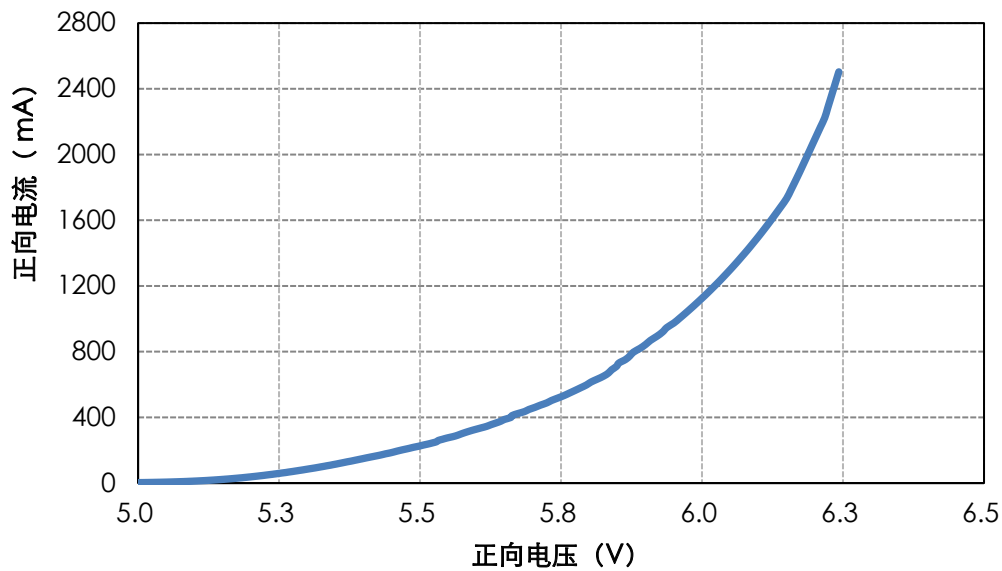
正向电压 vs 正向电流 (NLW7070P-F 6V, 环境温度25°C)
