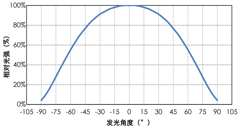
相对光强 vs 角度
