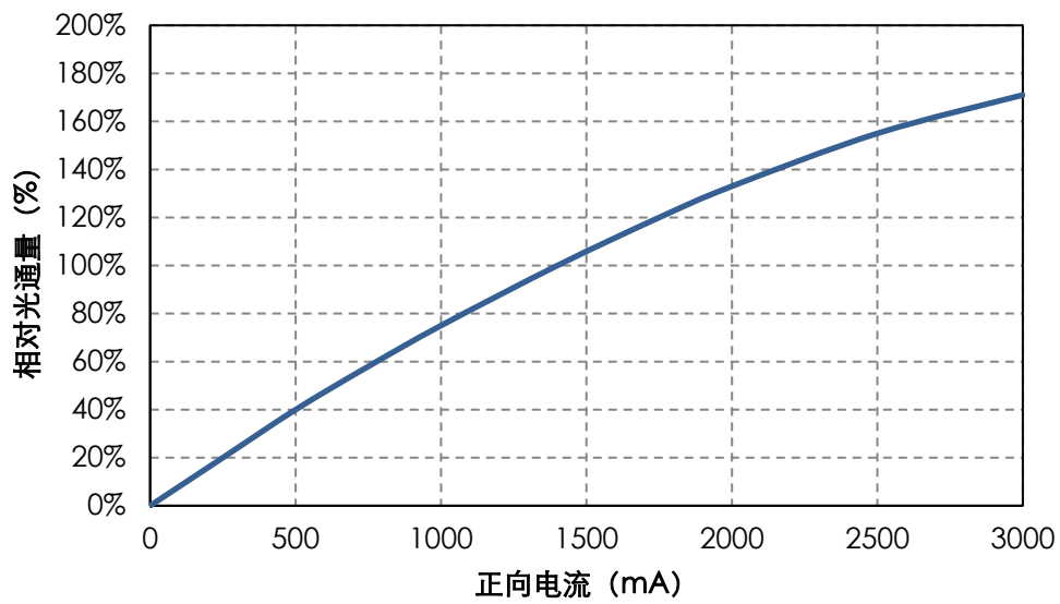
相对光通量 vs 正向电流 (测试时间20ms, 环境温度25°C)
