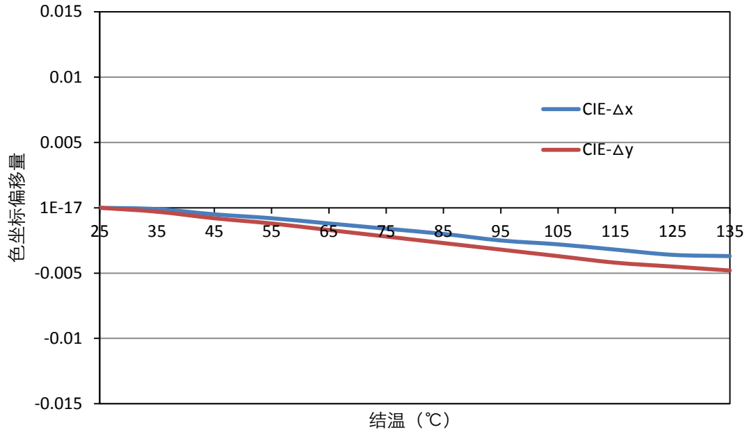
色坐标偏移 VS 结温
