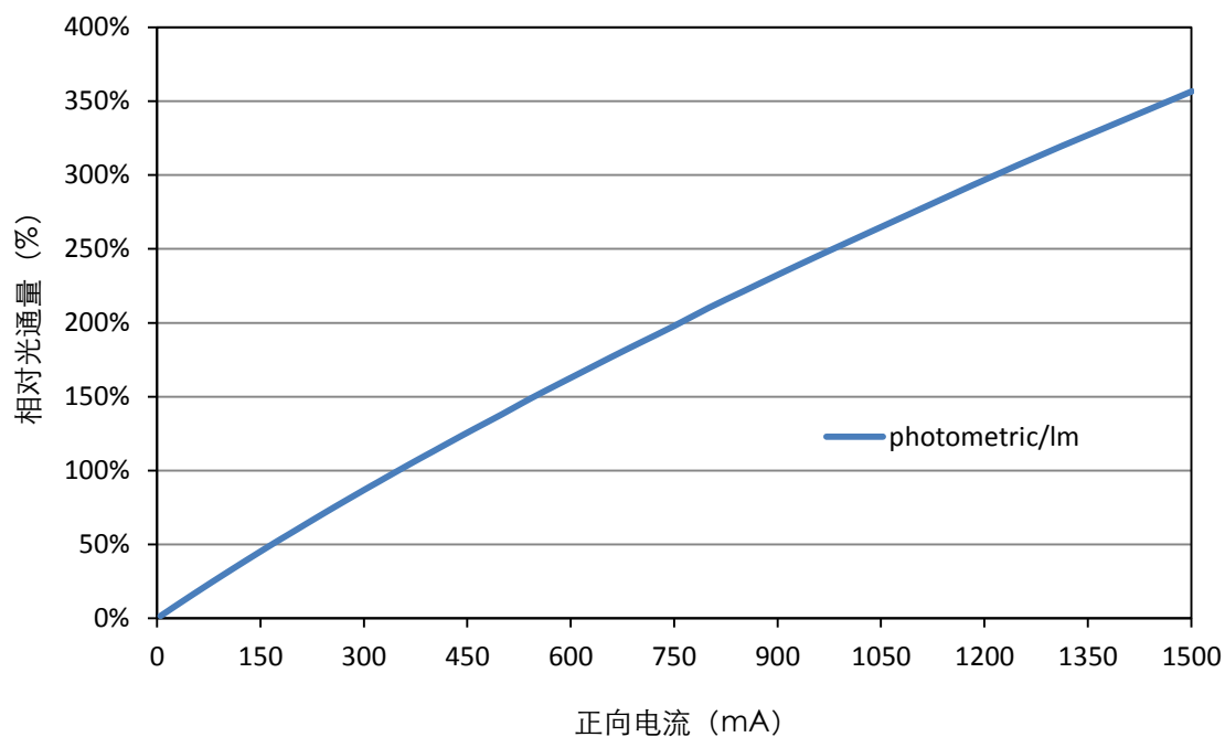
相对光通量 VS正向电流
