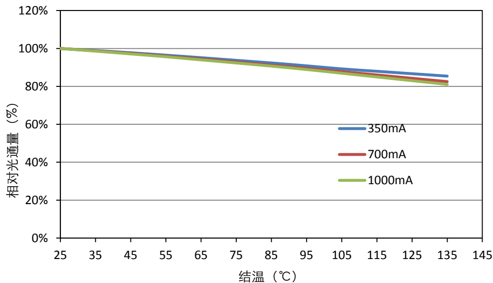
相对光通量 VS 结温
