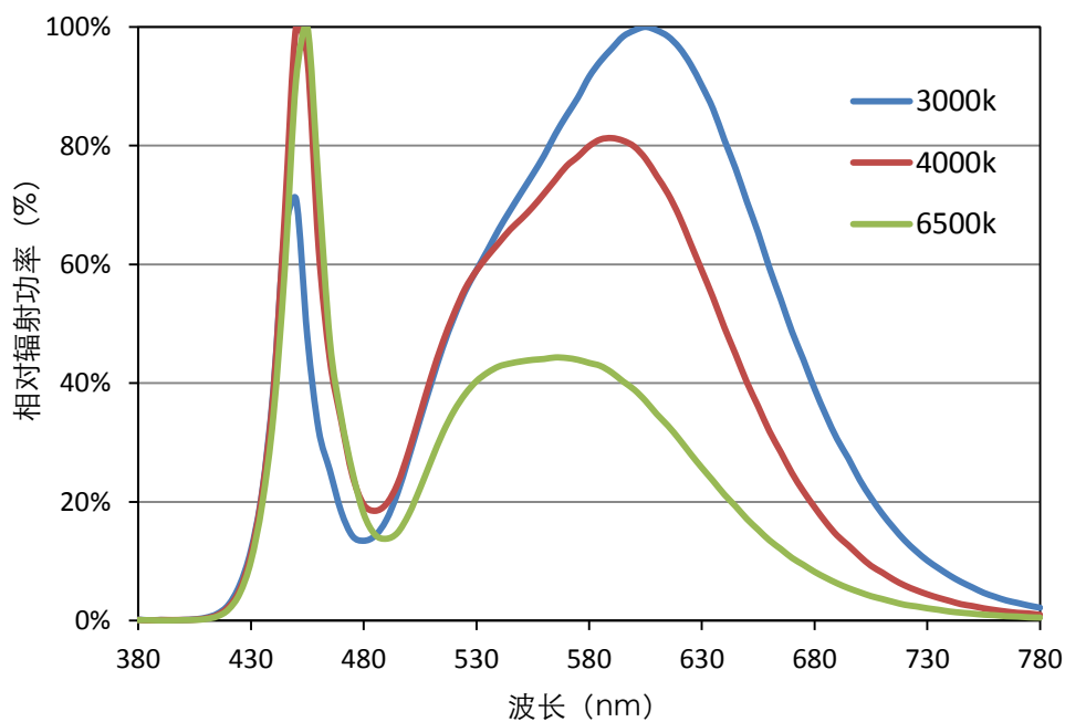
相对辐射功率 VS 波长
