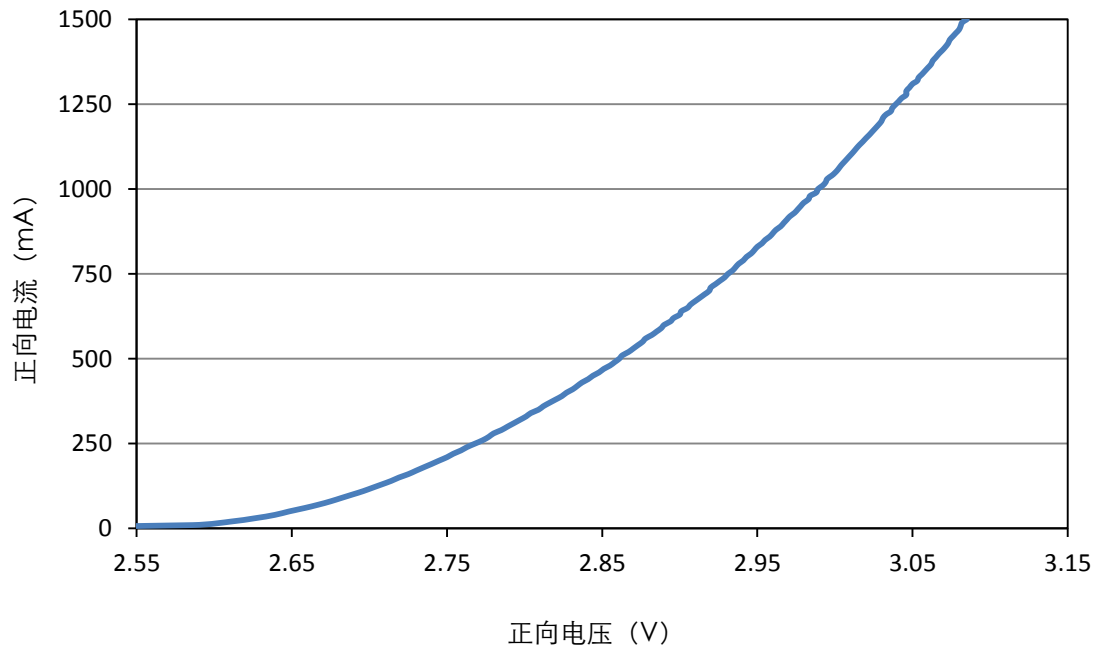
正向电流 VS 正向电压
